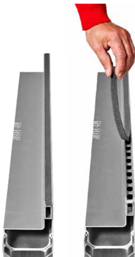
Alu Side Drain avec bande de protection
